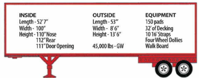
53' Air Ride Dry Van (Pad Wrap)
